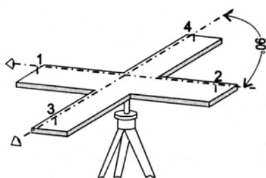
Slika 1: Kotni križ (Vir: Juvančič, 2000)
