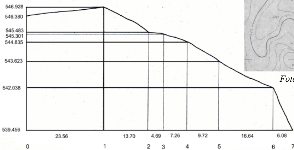
Slika 3: Podolžni profil terena (Vir: Anton Goršin)
