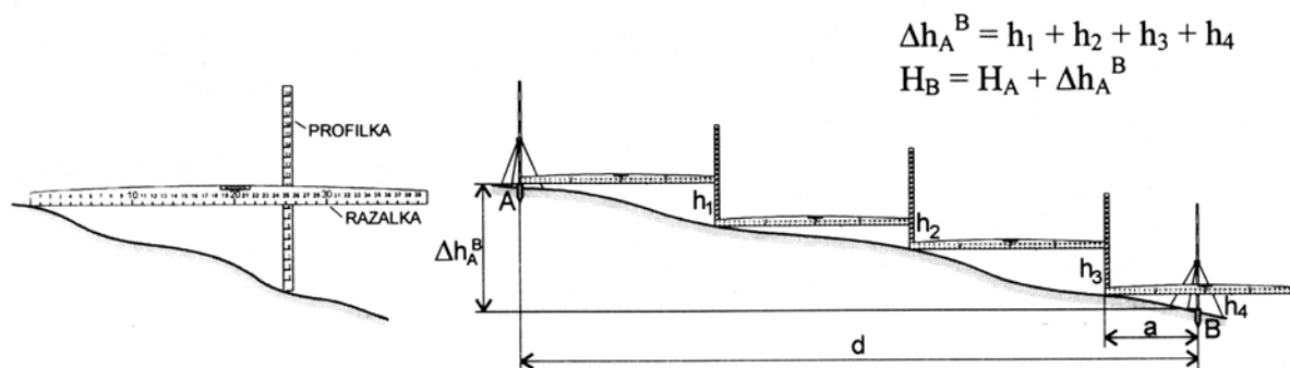
Slika 2: Potek izmere višinske razlike s postopičnim orodjem (Vir: Juvančič, 2000)
