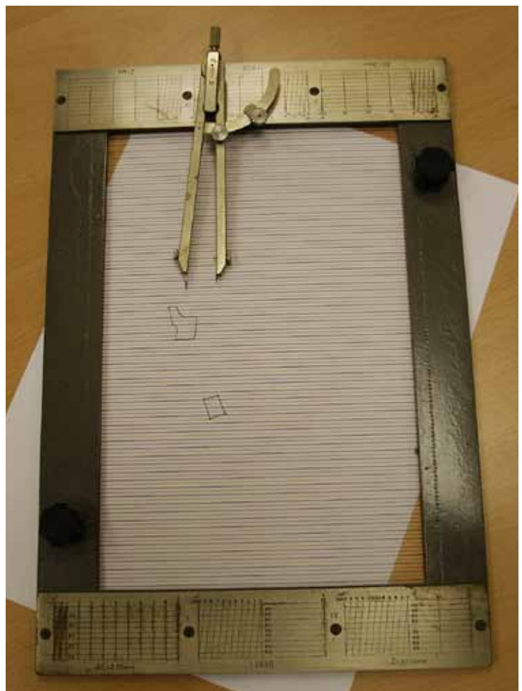
Fotografija 20: Planimeter za izmero površin (Vir: Anton Gorščin)
